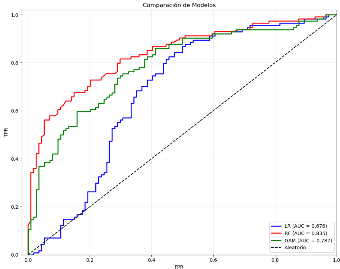
Figura 5. Evaluación comparativa del desempeño de modelos mediante análisis ROC. Comparación de Random Forest (AUC = 0.835, línea roja), (AUC = 0.787, línea verde), y Regresión Logística (AUC = 0.676, línea azul). Los métodos basados en datos superaron consistentemente a los enfoques heurísticos.
