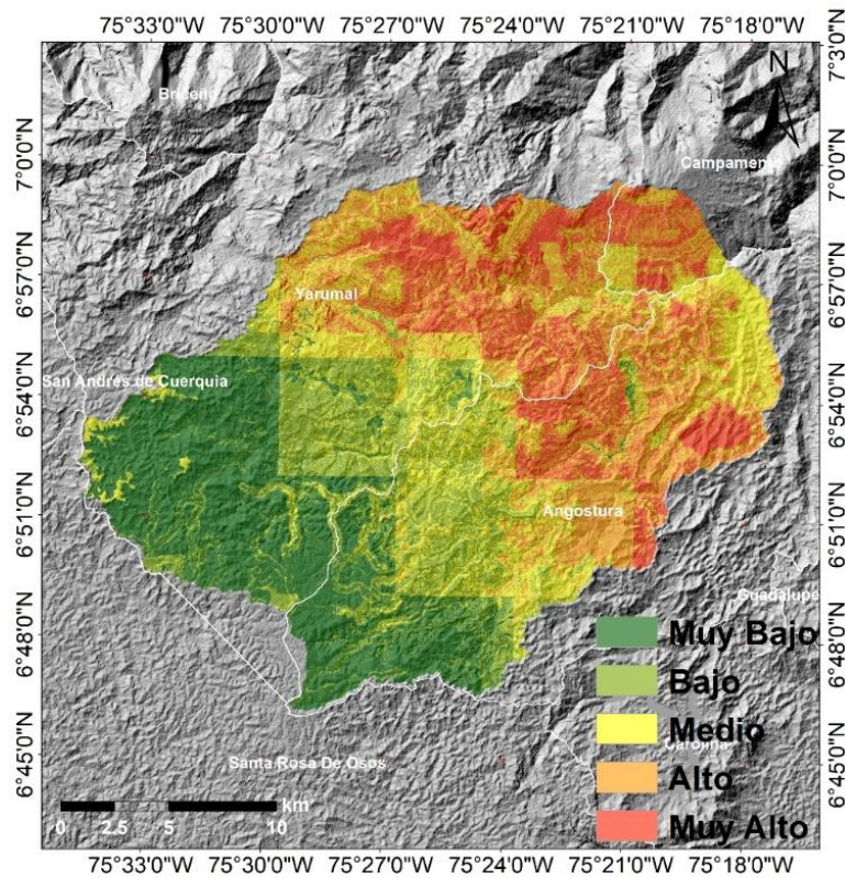
Figura 8. Zonificación integrada de amenaza combinando susceptibilidad espacial y análisis de precipitación. Combinación matricial de Random Forest con factor lluvia clasificado por tipo de material. Cinco categorías de amenaza con concentración en laderas de alta pendiente del Batolito Antioqueño.
